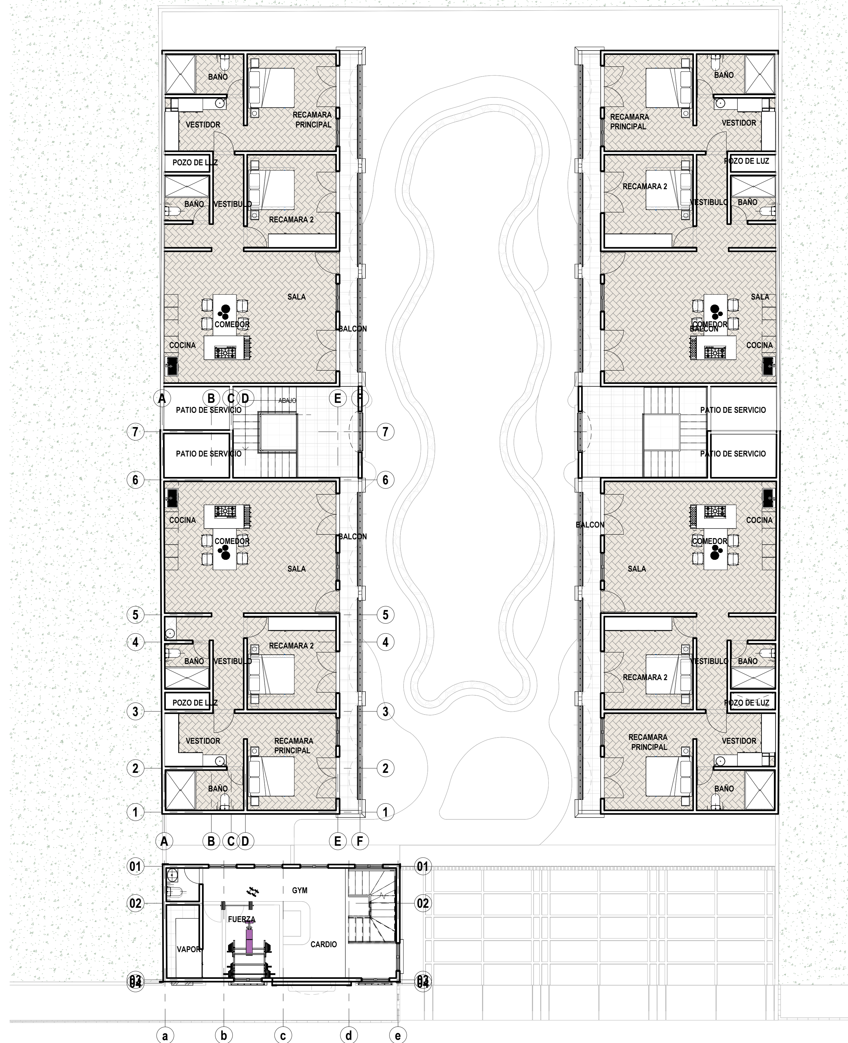
2 01. Planta alta+ 3.06mts 1 : 100
