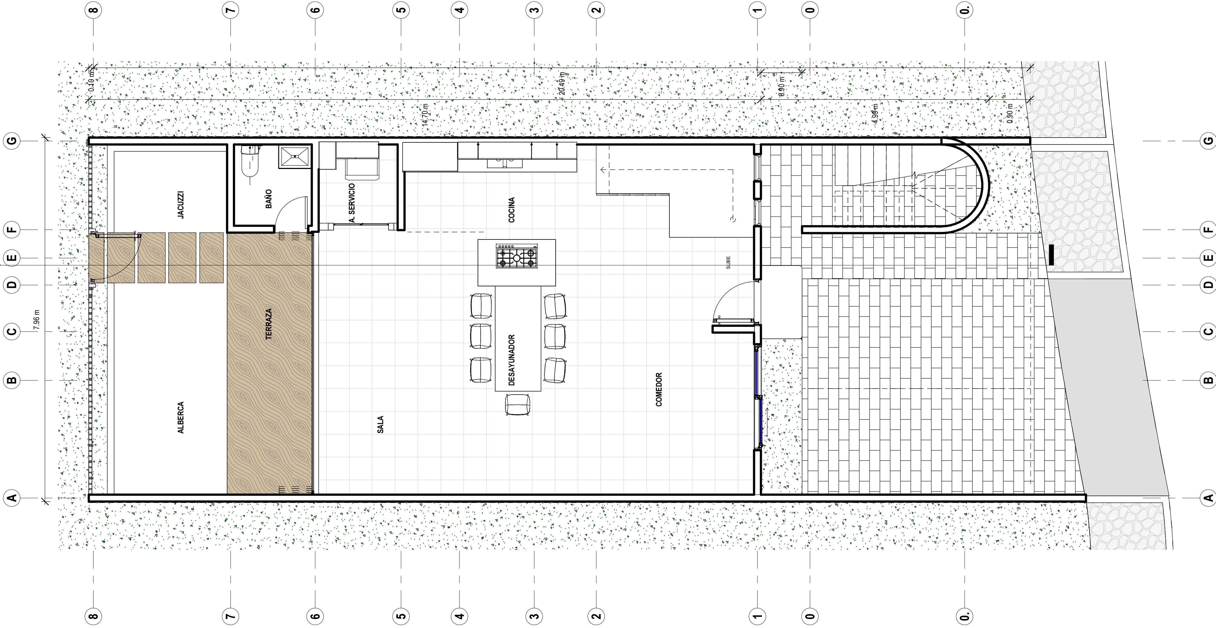
1 0.2. Planta baja +0.34mts
